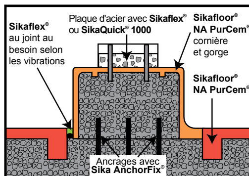
SOCLE DE MACHINE
