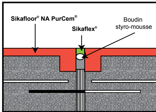
JOINT DE CONTRÔLE/DILATATION
