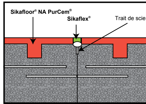
JOINT AU SOL
