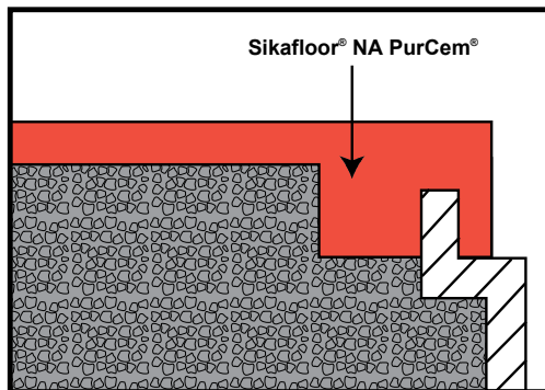
BORD DE DRAIN ÉMAILLÉ
