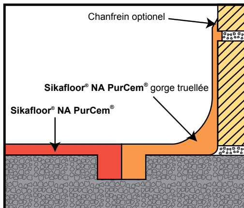
PLINTHE À GORGE ET MURËT
