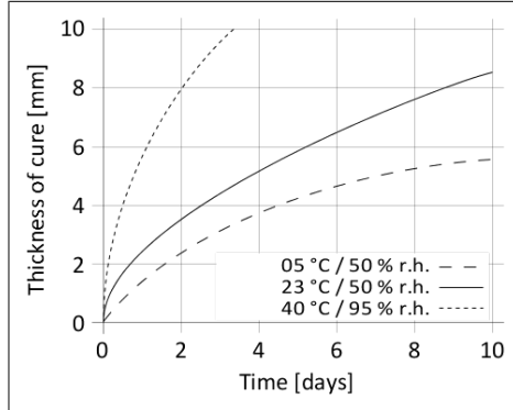
Diagramme 1 : Vitesse de mûrissement du Sikasil® WS-304 ME
