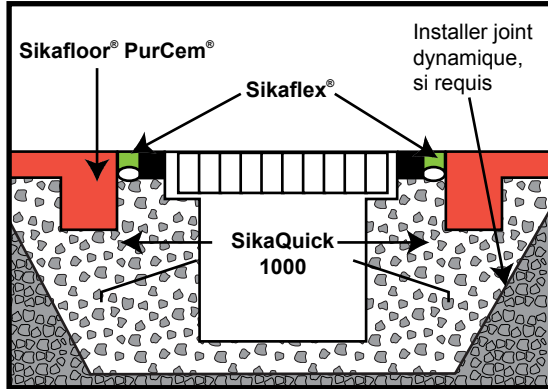
Sikafloor® PurCem® – Caniveau préformé
