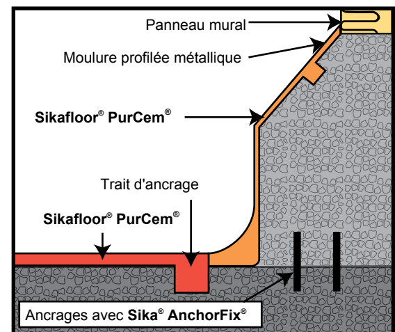
Sikafloor® PurCem® – Détail d'une bordure
