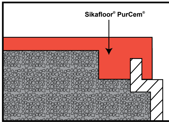
Sikafloor® PurCem® – Bord de drain émaillé
