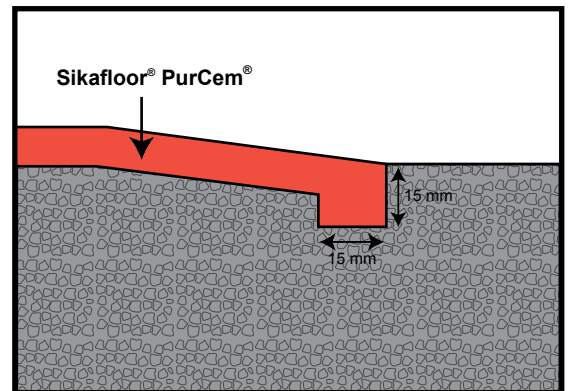
Sikafloor® PurCem® – Épaisseur au bord
