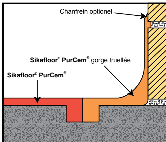
Sikafloor® PurCem® – Plinthe à gorge et murêt
