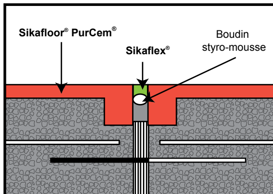
Sikafloor® PurCem® – Joint de contrôle/dilatation
