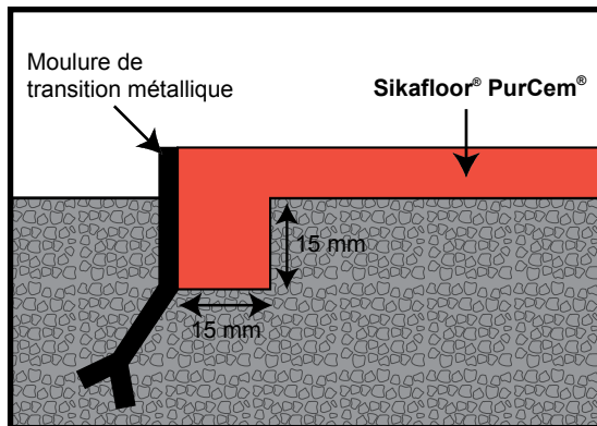
Sikafloor® PurCem® – Extrémité métallique
